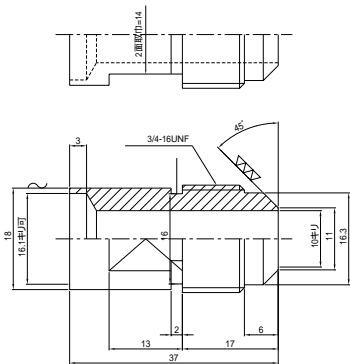
ニップル詳細図
