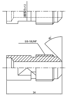
ニップル詳細図
