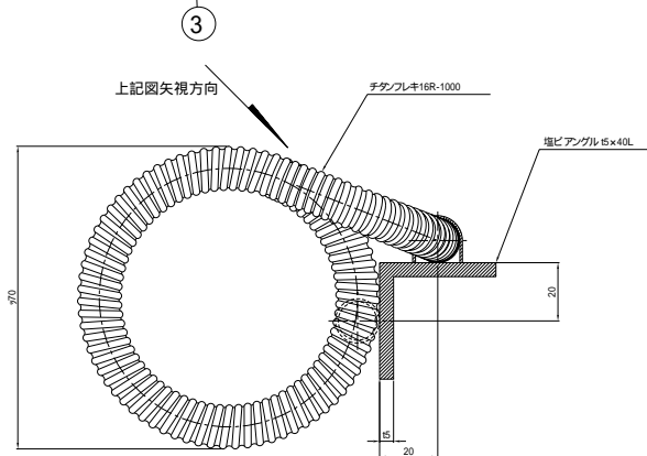
アングル部詳細(尺度1/2)
